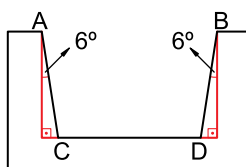
Vista frontal do corte transversal feito no molde
