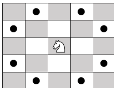
Figura 1 – Possibilidades de movimentação do cavalo
